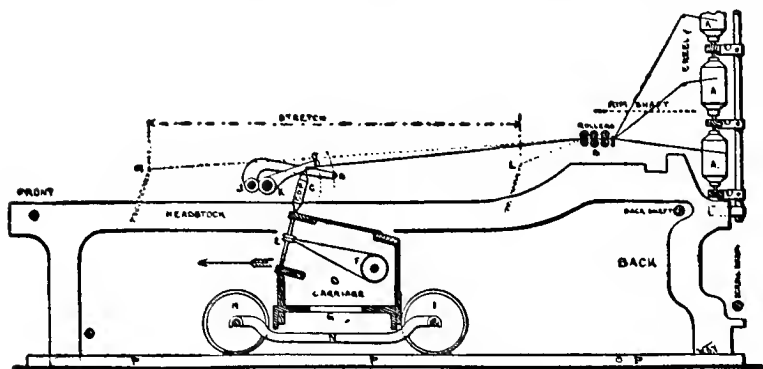
FIG. 4. CROMPTON'S MULE
